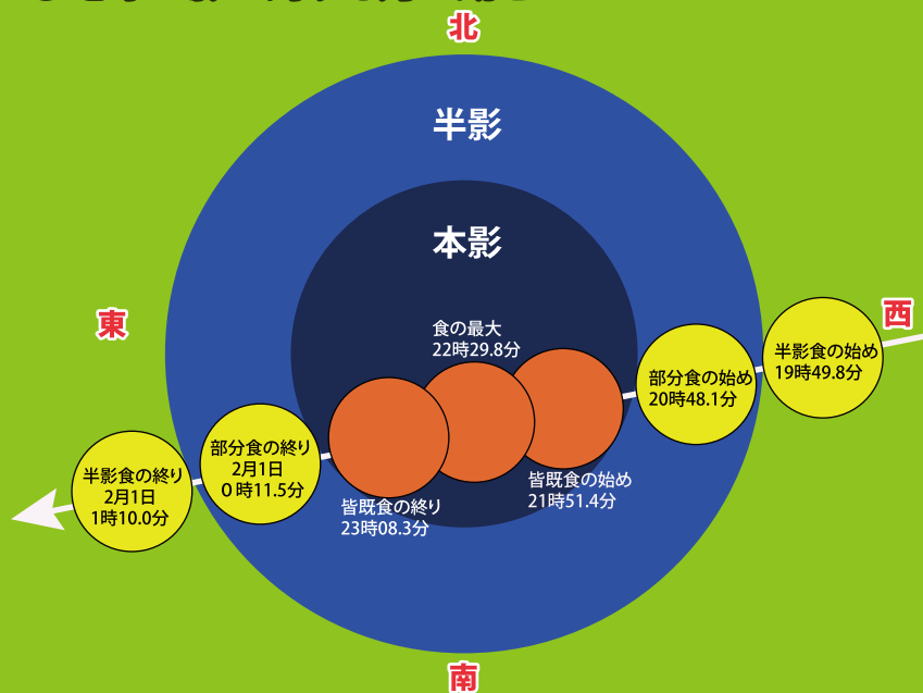
◎地球の影に対する月の動き
